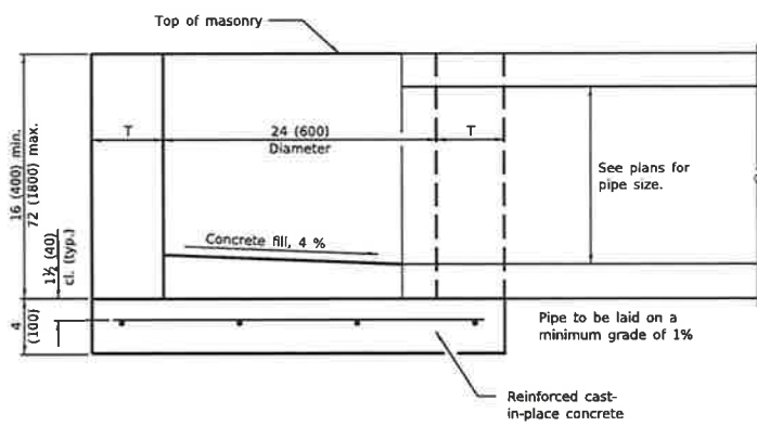
ELEVATION
